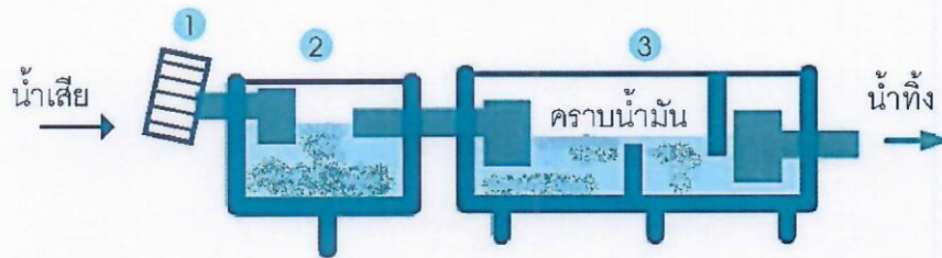
รูปที่ ๕ บ่อดักและบ่อดักไขมันสถานีบริการน้ำมันเชื้อเพลิง
